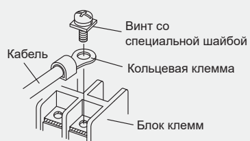
Многожильный гибкий кабель
