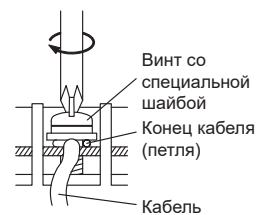
Одножильный твердый кабель
